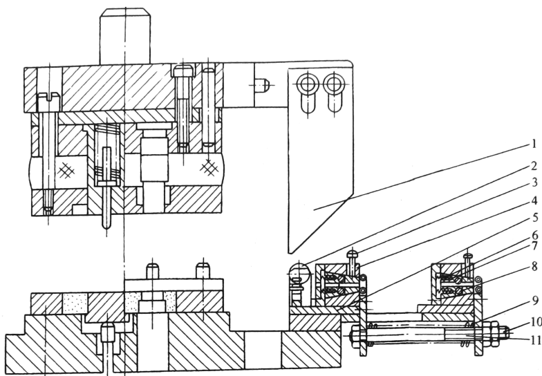
1—斜楔; 2—滑轮; 3—拨杆; 4—外座; 5—滚柱座; 6—弹簧; 7—保持架; 8—滚柱; 9—弹簧; 10—螺母; 11—螺杆 题 27 图
